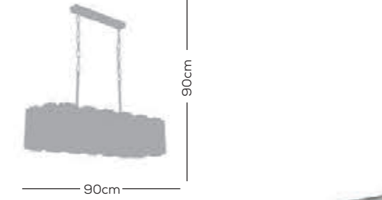
Kod: LRZ 555-90-YM-AB 7 x E14 Max 40W
